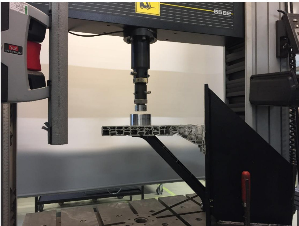
Billede 2. Samme opstilling set fra side – bemærk placering af punktblast i centrum af stiverens fastgørelsespunkt.
