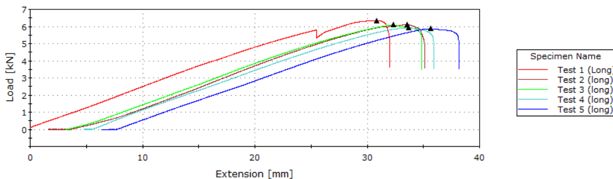
Billede 3: Resultater af bæreevnetest for stor skrånstiver
