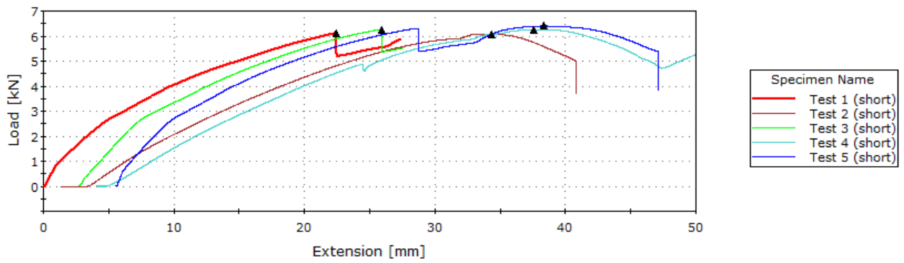
Billede 4: Resultater af bæreevnetest for lille skråstiver
